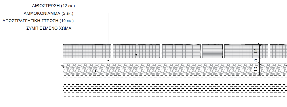
ΤΟΜΗ ΚΛ.:1/20
